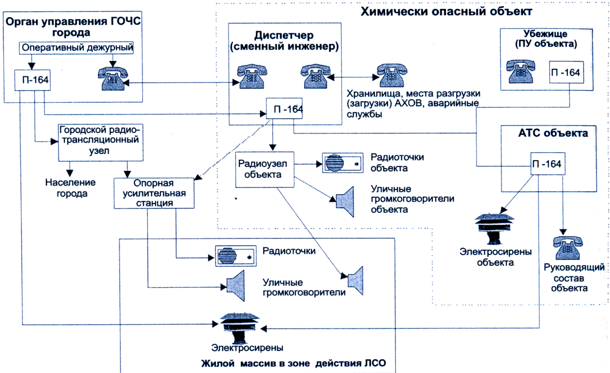
Схема построения ЛСО химически опасного объекта
